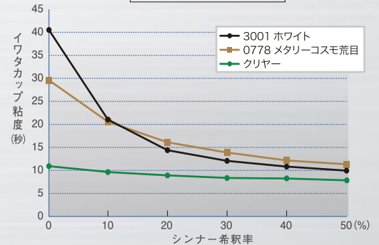
希釈粘度曲線
