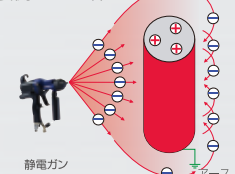
静電ガン
