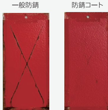
※JIS K5600-7-1 塩水噴霧試験(1000時間)
